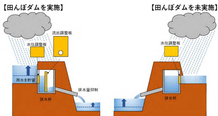
図7-4 「田んぼダム」のイメージ
