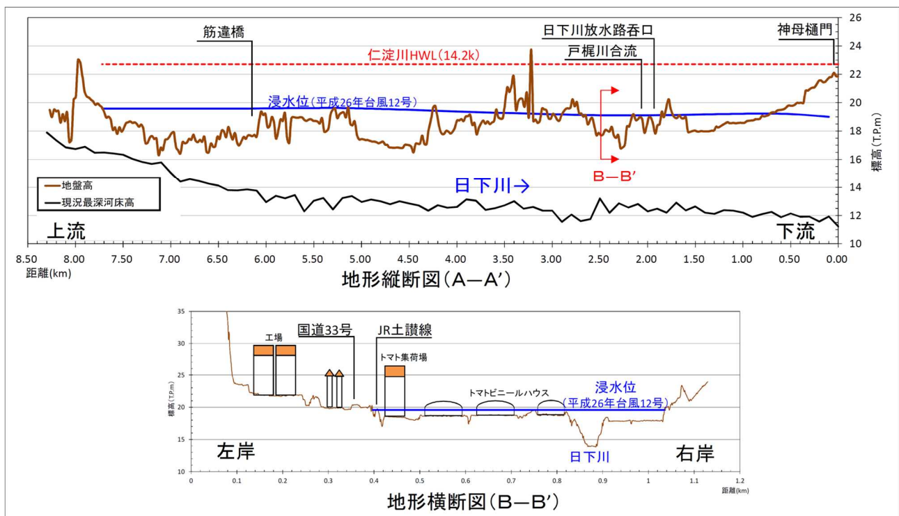
図1-12 日下川特定都市河川流域の堤内地の状況
