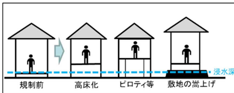
図9-3 建築物の浸水対策のイメージ
