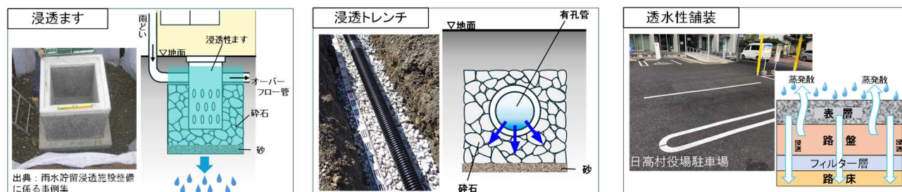
図8-1 雨水貯留浸透施設の例
