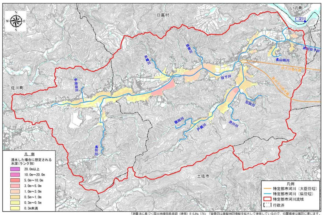
図10-2 ハード整備実施後の都市浸水想定区域図
