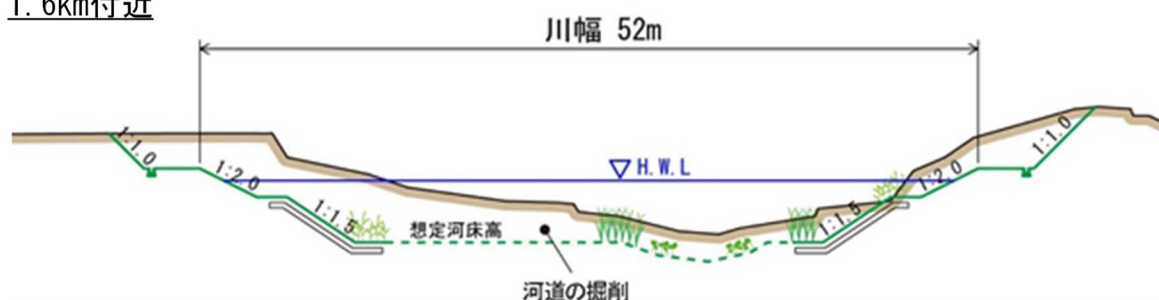
図4-3 目下川の整備イメージ
