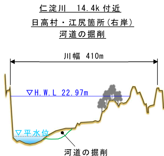
図4-1 河道の掘削等イメージ
