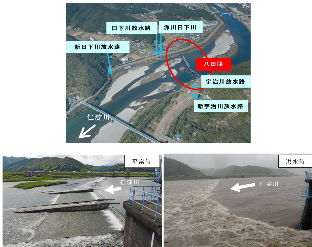
図4-2 八田堰の位置、平常時及び洪水時の状況
