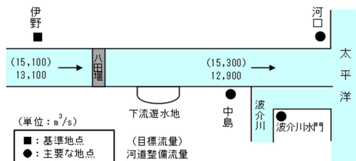
図1-19 河道整備流量配分図
