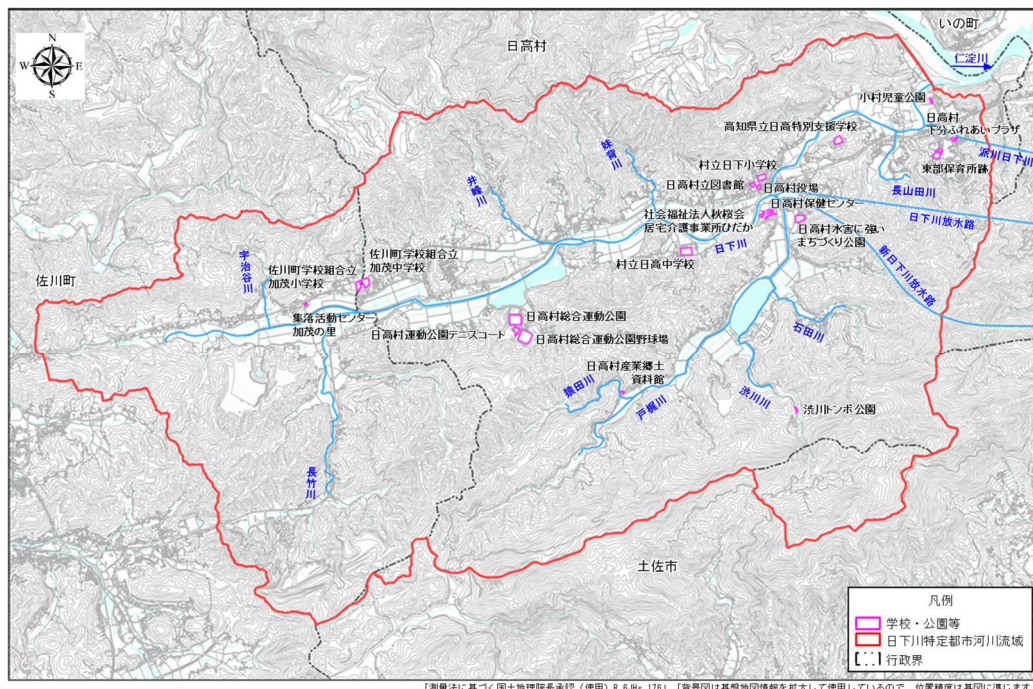
図7-1 雨水貯留施設の整備候補地（学校・公園等）の配置状況
