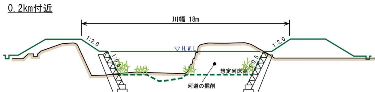
図4-5 長竹川の整備イメージ
